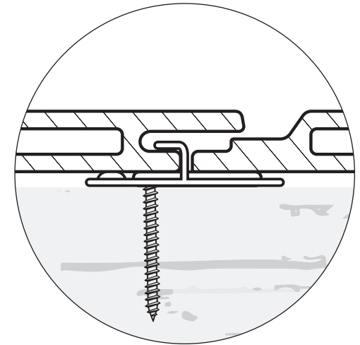
Befestigung per Clip
