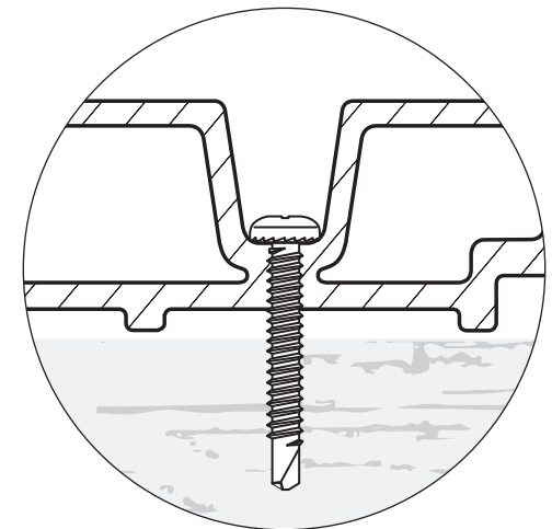
Befestigung per Schraube
