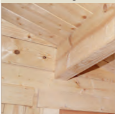
Dachpfetten 70x180 mm; Dachbelastbarkeit über 180 kg/m 2
