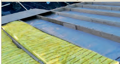
Detail: Abb. 44/70 mm Bohle
