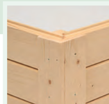
Steck-Schraub-Variante 28 oder 40 mm Bohle
