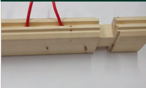
inkl. Bohrungen für Elektroleitung des Saunaofens
